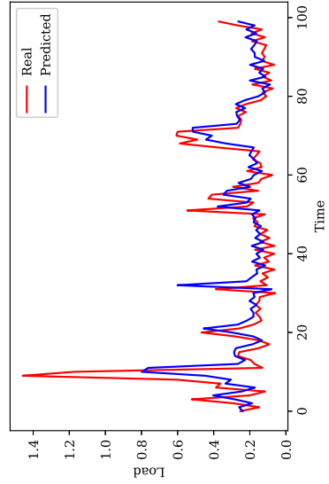
d) GRU
