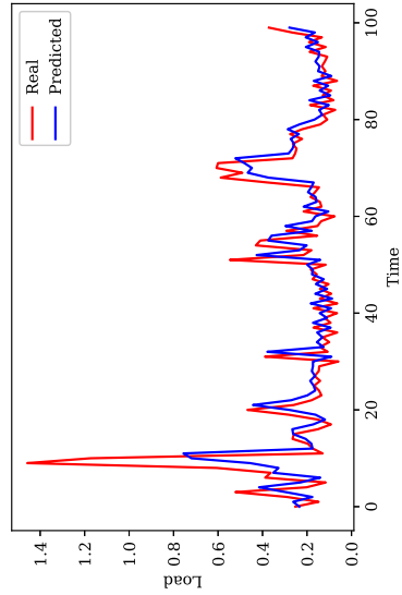
f) LightGBM
