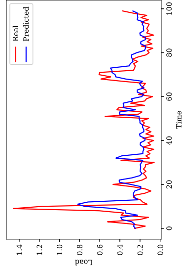
b) CNN-LSTM
